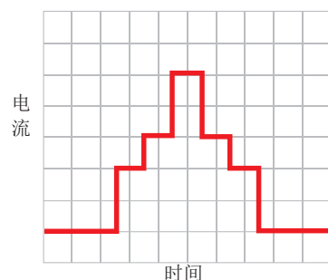
图2 - 模块的序列
