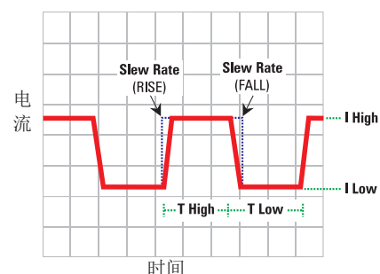
图4 - 直流型号动态模式
