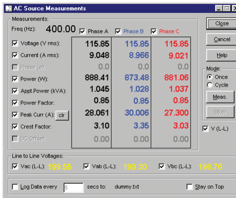
所有相位的标准测量
