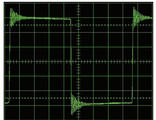
在UPS输出上猛烈振铃的模拟。
